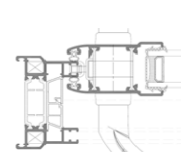
Jamb Detail
